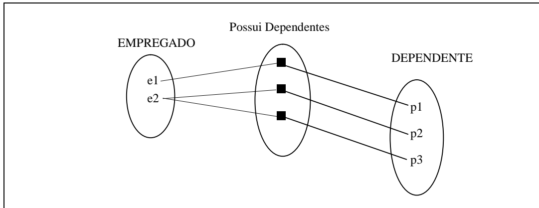
Figura 9 - Relacionamento com uma Entidade Fraca (Dependente)
