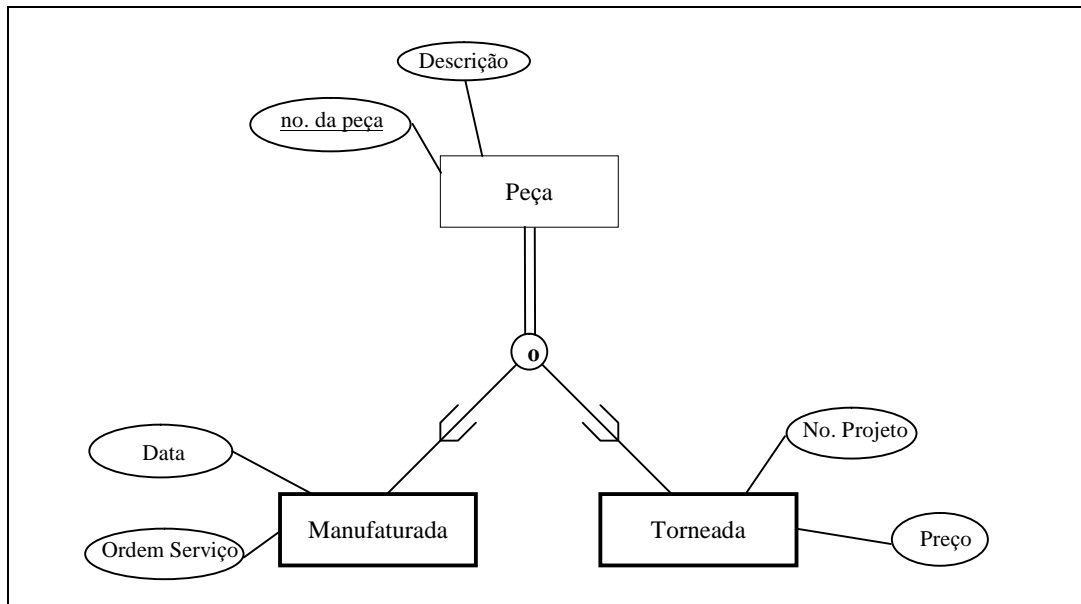
Figura 17 - Uma Generalização com “Overlap”
