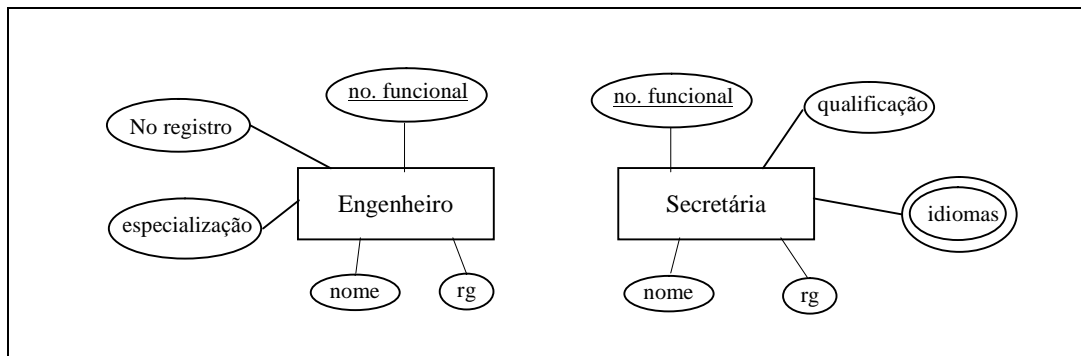
Figura 15 - Tipos Entidades Engenheiro e Secretária
