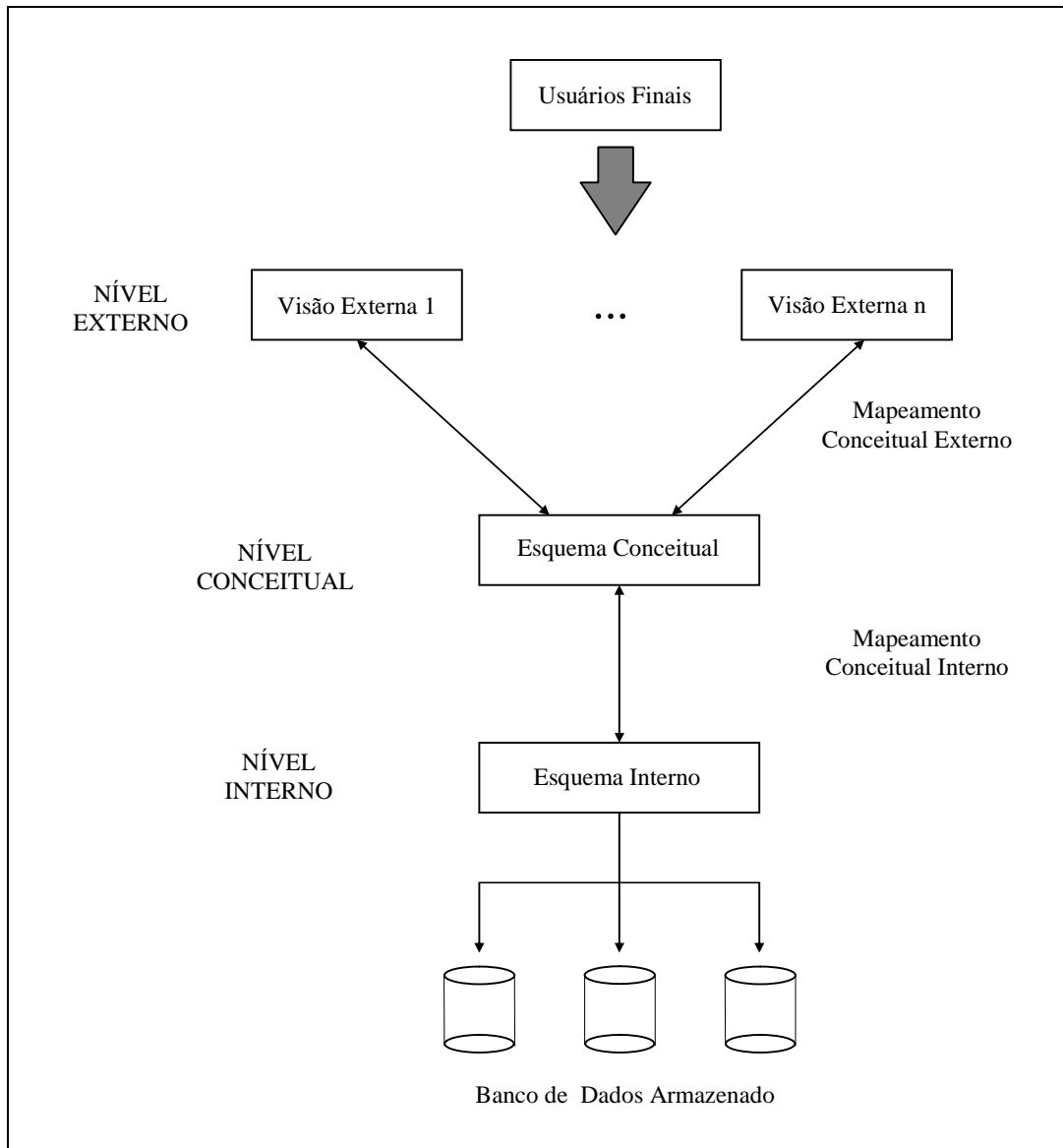
Figura 2: Arquitetura Três Esquemas
