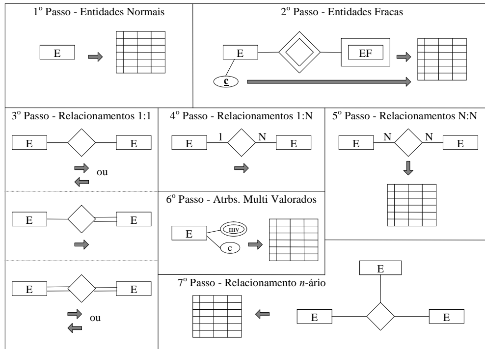
Figura 19 - Mapeamento para o Modelo Relacional
