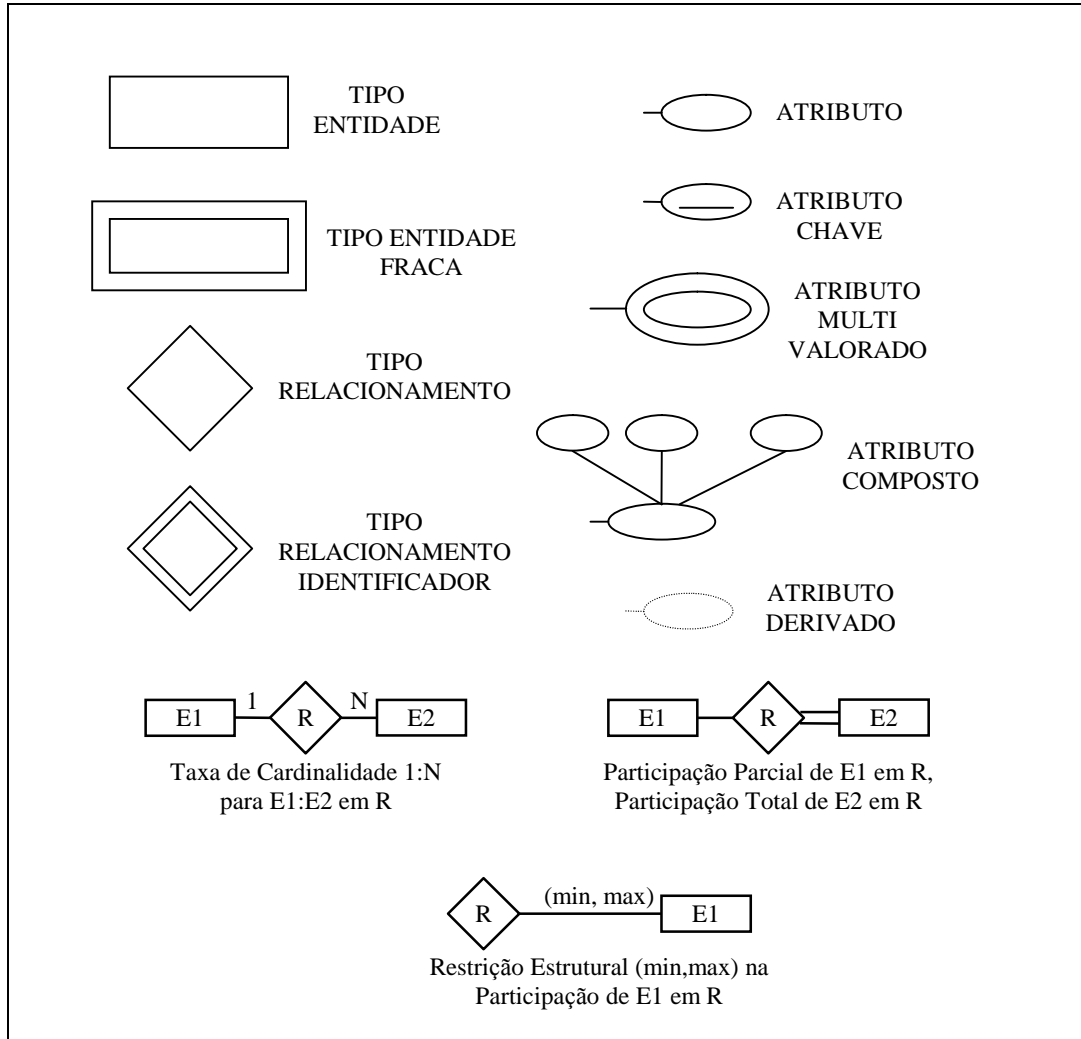
Figura 11- Objetos que Compõem o Diagrama ER
