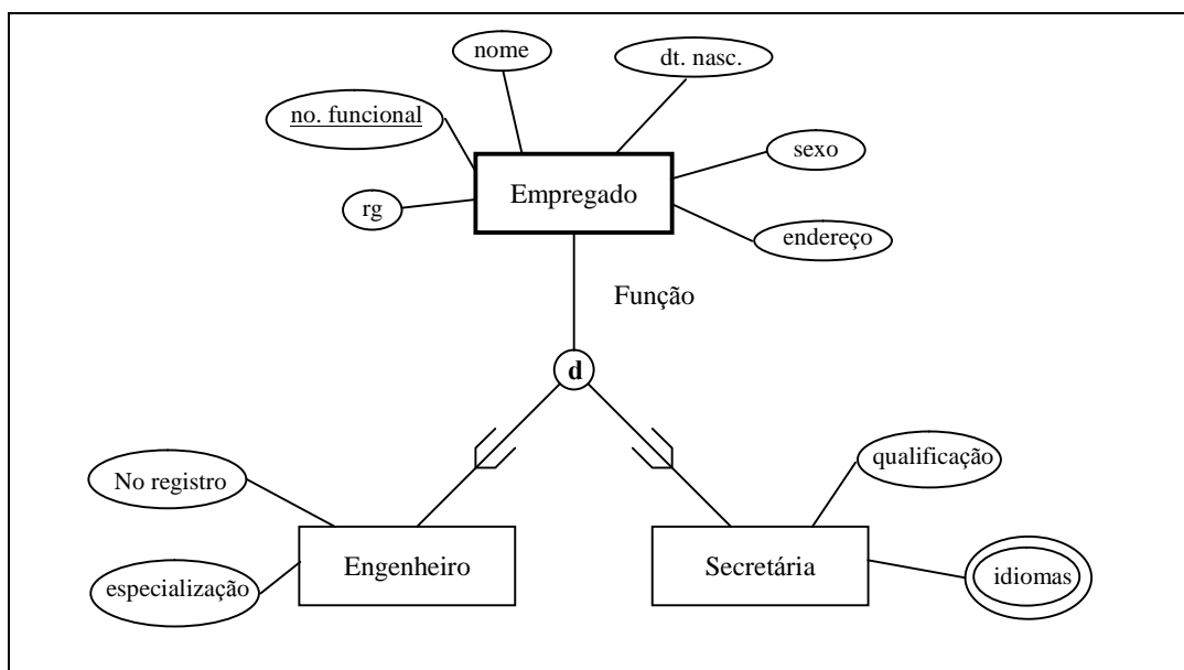
Figura 12 - Representação de Superclasse e Subclasses
