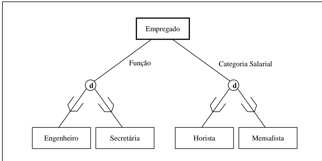
Figura 13 - Duas Especializações para Empregado: Função e Categoria Salarial
