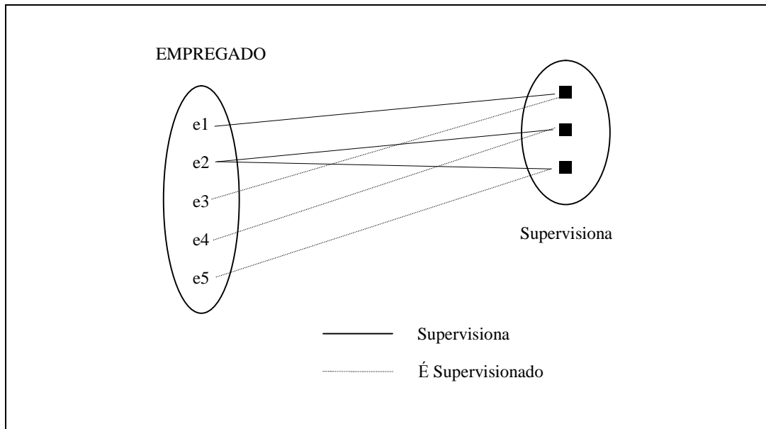
Figura 6 - Um Relacionamento Recursivo
