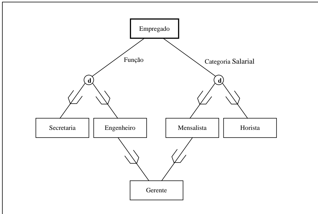
Figura 18 - Um “Lattice” com a Subclasse Gerente Compartilhada
