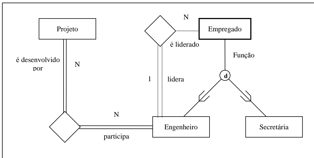
Figura 14 - Relacionamentos Entre Subclasses e Entidades
